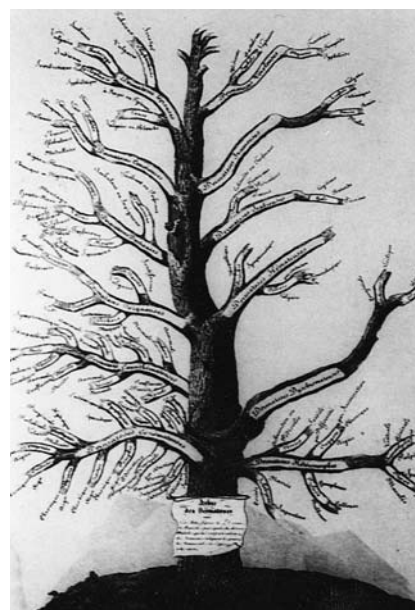
Fig. 2.—Arbre des dermatoses de Alibert.
